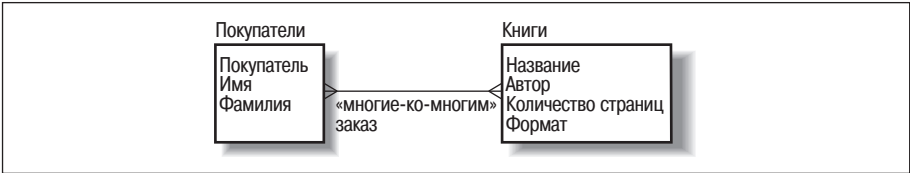
Рис. 8.5. Связь «многие-ко-многим» между покупателями и приобретенными книгами
