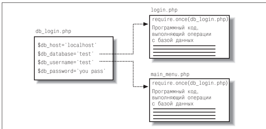
Рис. 9.2. Использование информации о подключении к базе данных в нескольких сценариях
