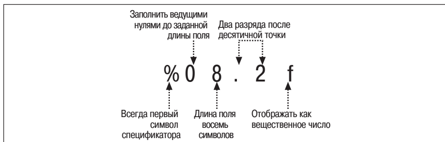
Рис. 11.9. Составные части спецификатора формата
