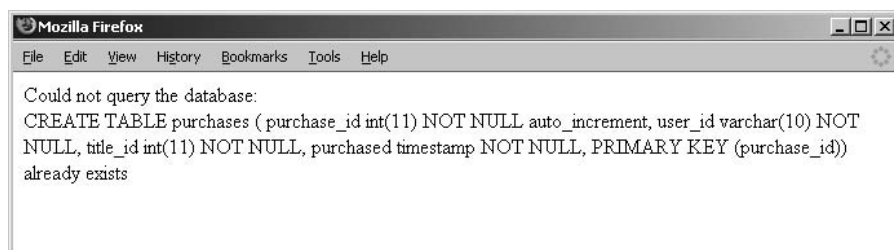
Рис. 13.2. При попытке создать существующую таблицу появляется такое сообщение
