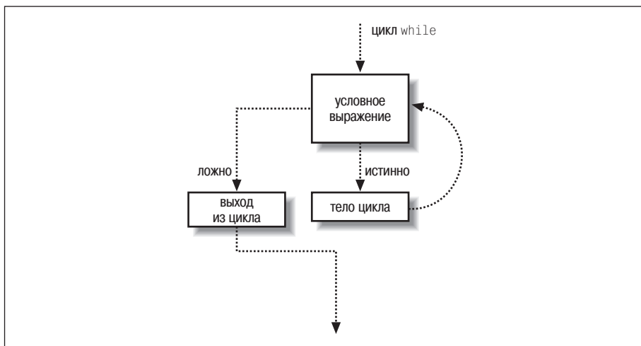
Рис. 4.3. Так выполняется цикл while
